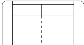
Manu 2P W:1760 D:960 H:810 SH:440
