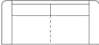
Manu 3P W:2110 D:960 H:810 SH:440
